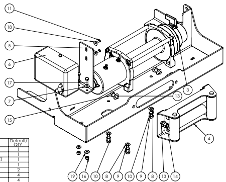
WINCH FRAME 301010212 ARBTRAK 190 & 200
