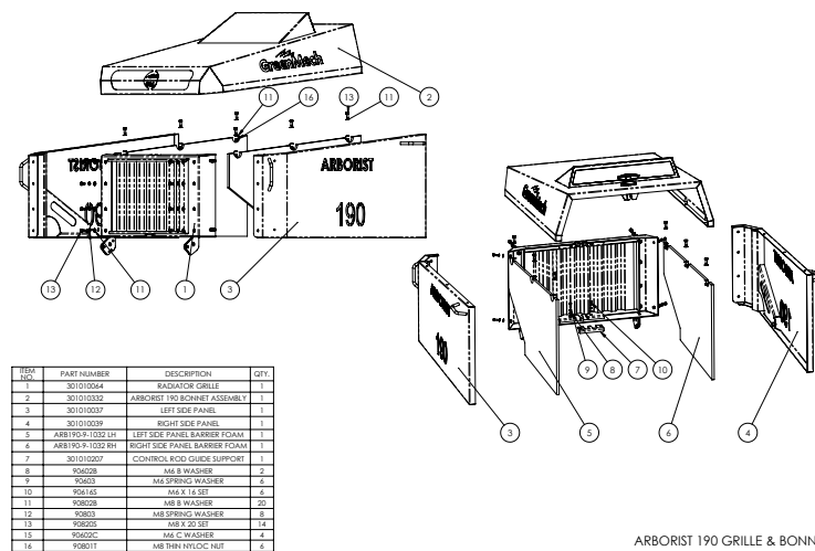
ARBORIST 190 GRILLE & BONNET 301010331
