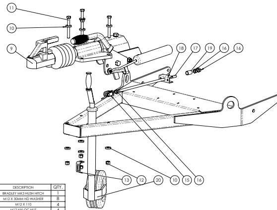
A FRAME 301010048 ARBORIST 190 & 200
