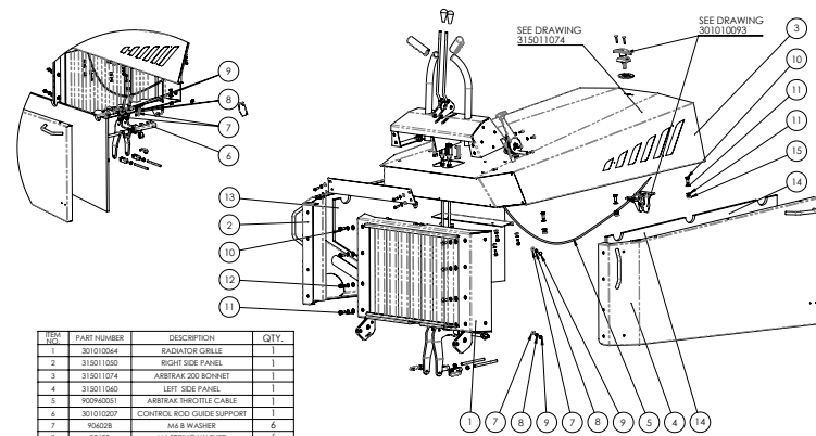
ARBTRAK 200 GRILLE & BONNET 315011055
