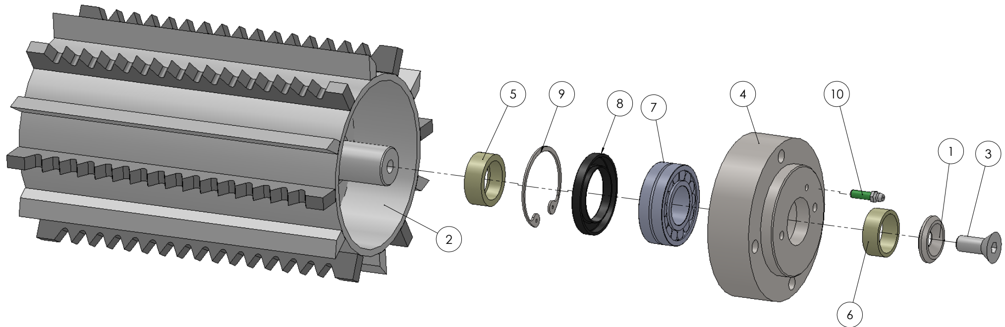
BOTTOM ROLLER
